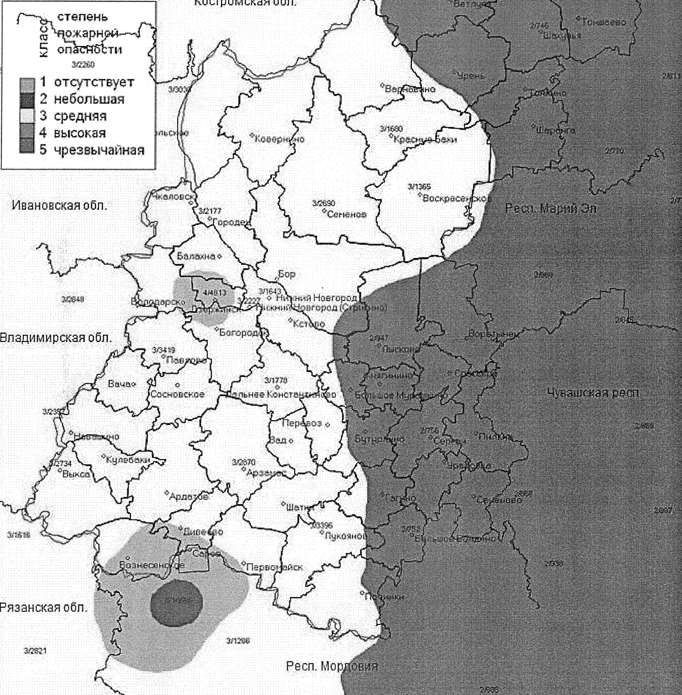
Карта пожароопасности Нижегородской области в числителе-класс, в знаменателе-показатель горимости на 12 час. ВСВ 01 июля 2026 года
